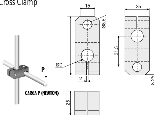
Mordaza En Cruz Cross Clamp
